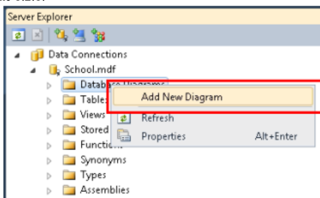
Рисунок 1.2.1 Добавление диаграммы
